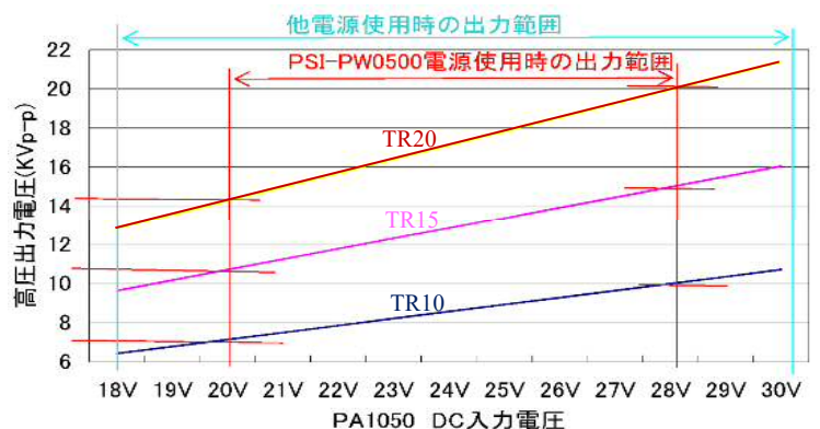
Fig 1: PA1050(パワーアンプ)-TR**(高電圧トランス出力)
